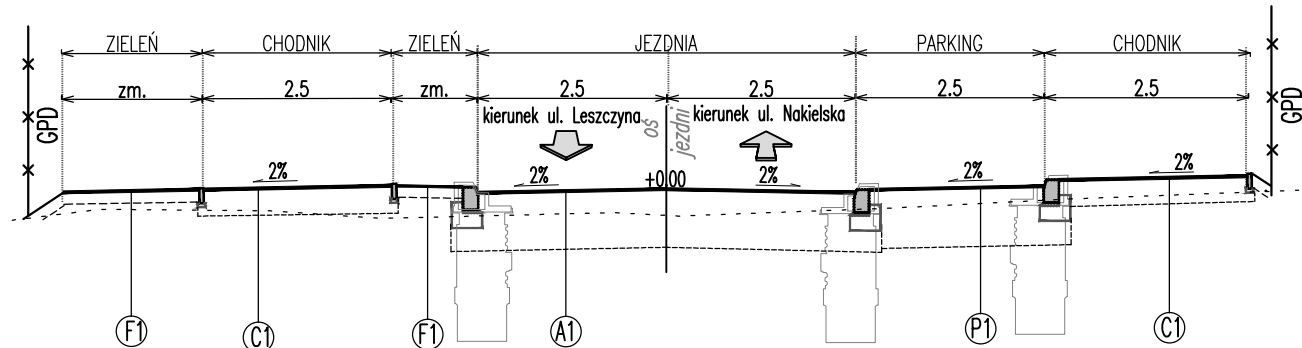
PRZEKRÓJ NORMALNY 2 – B-B
