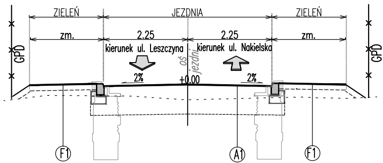
PRZEKRÓJ NORMALNY 6 – F-F
