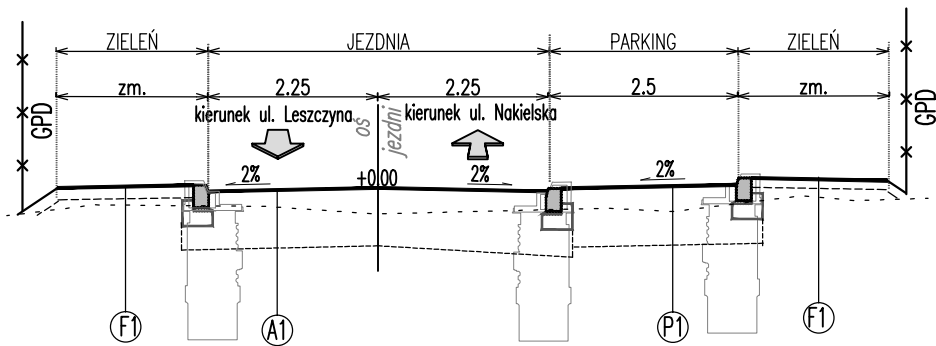
PRZEKRÓJ NORMALNY 3 – C-C
