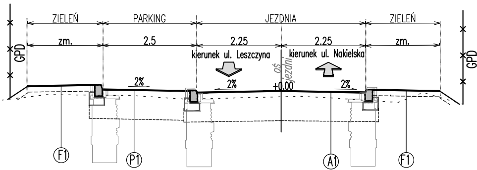
PRZEKRÓJ NORMALNY 4 – D-D
