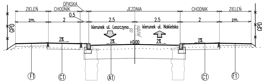
PRZEKRÓJ NORMALNY 1 – A-A
