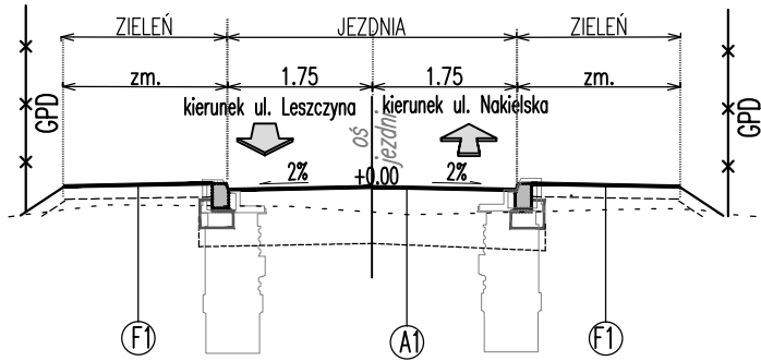
PRZEKRÓJ NORMALNY 5 – E-E
